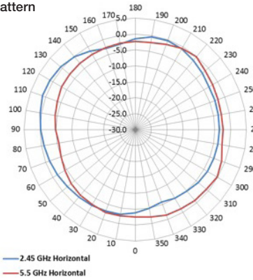
H-Plane Pattern
