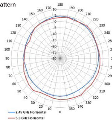
H-Plane Pattern
